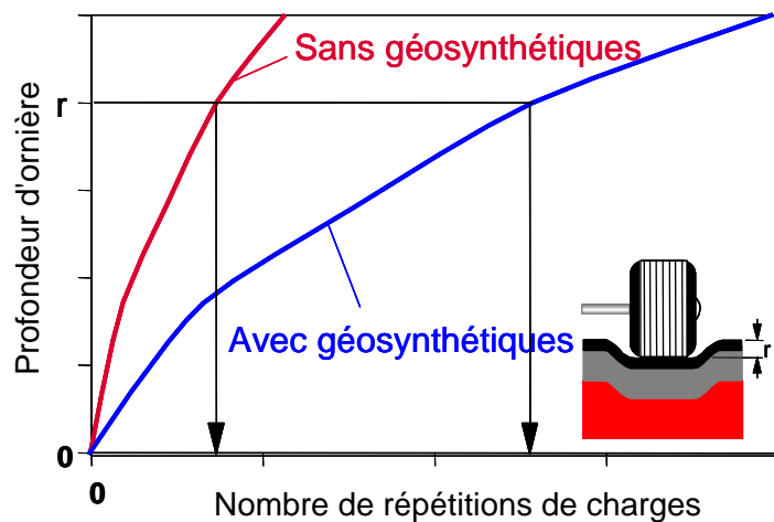
Augmentation de la durée de vie de la chaussée en lien avec l'utilisation d'un renforcement géosynthétique
